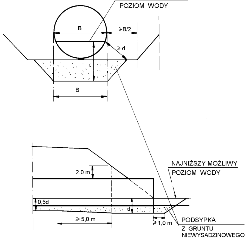
Rys. 6. Sposób wykonania podsypki pod przepustem, posadawianym na gruncie wysadzinowym NAJNIŻSZY MOŻLIWY POZIOM WODY
