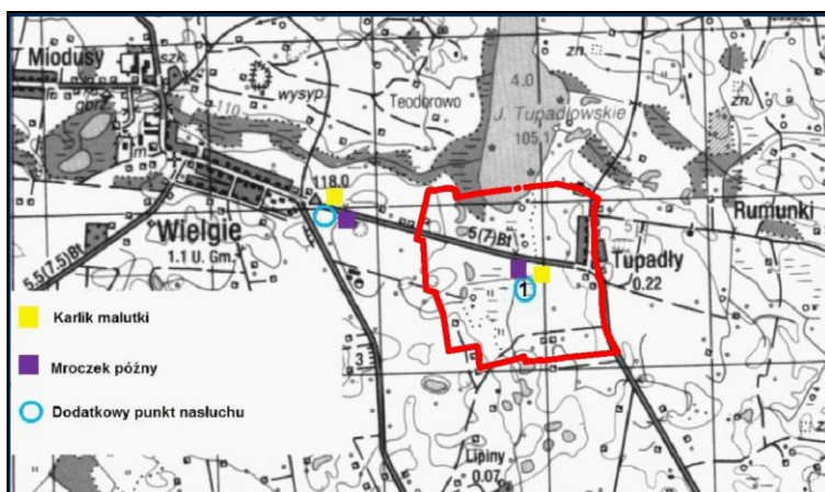
Rys. 3. Stwierdzenia aktywności gatunków nietoperzy w monitorowanych punktach (okolice m. Wielgie i Tupadły) w okresie tworzenia kolonii rozrodczych i rozrodu w obrębie obszaru opracowania
