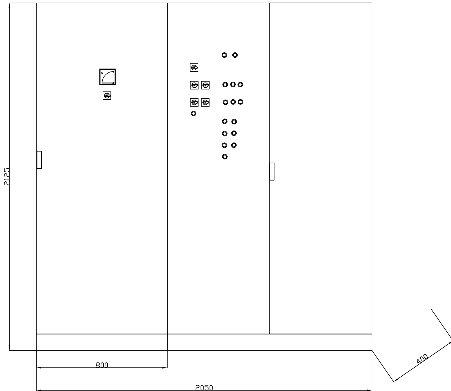
Rozdzielnica RG - SUW 0rtowo 0budowa typu SVTL IP54
