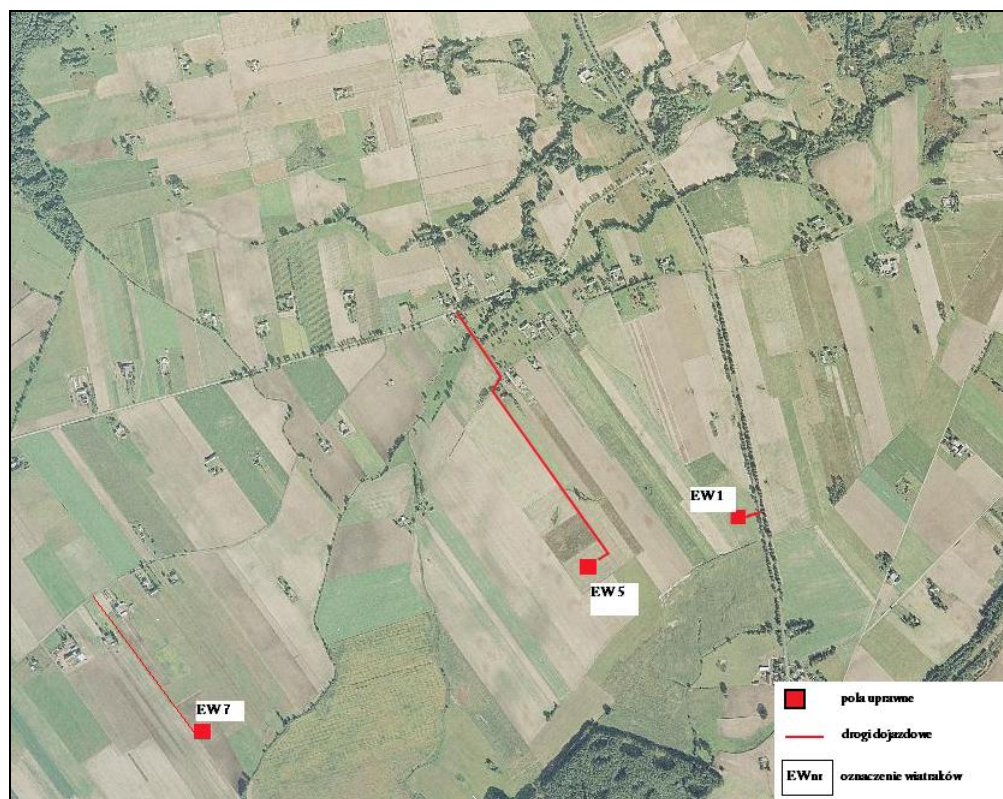
Rys. 1. Ortofotomapa z wyszczególnieniem chronionych siedlisk i gatunków roślin na terenach lokalizacji elektrowni wiatrowej E1 i E5.
