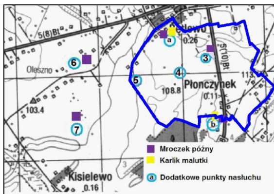
Rys. 4. Stwierdzenia aktywności gatunków nietoperzy w monitorowanych punktach (okolice m. Bętlewo i Płoczynek) w okresie tworzenia kolonii rozrodczych i rozrodu w obrębie obszaru opracowania (linia niebieska)
