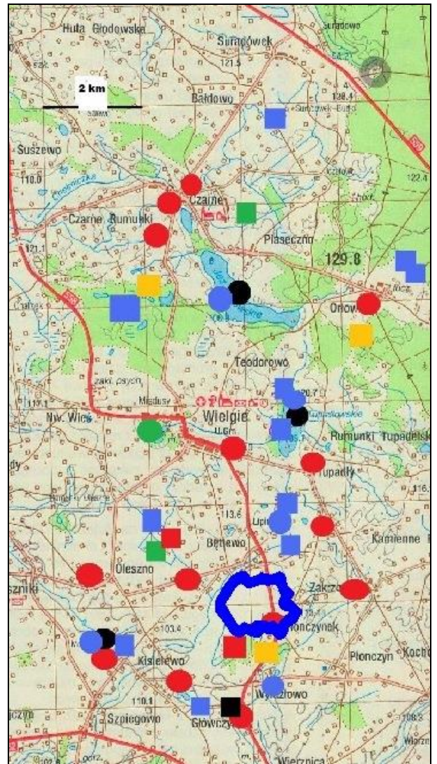
Rys. 3. Rozmieszczenie stanowisk lęgowych gatunków niewróblowych z Załącznika 1 tzw. dyrektywy ptasiej w obrębie terenu opracowania (linia niebieska). Koła: czerwone (bocian biały), czarne (bąk), zielone (trzmielojad), niebieskie (błotniak stawowy). Kwadraty: czerwony (dzięcioł średni), żółty (dzięcioł czarny), niebieski (żuraw), czarny (błotniak łąkowy), zielony (derkacz). Źródło: Cisakowski R., (2010)
