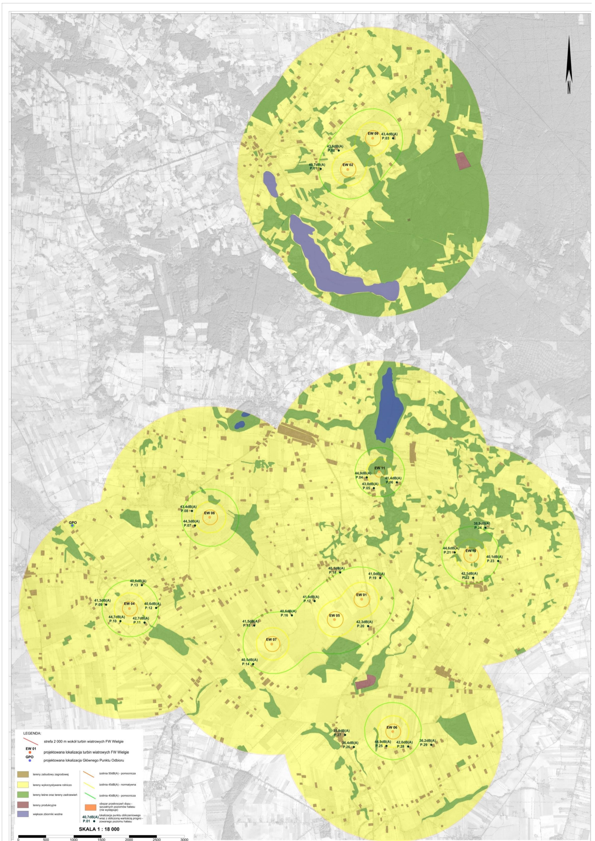
Rys. 8. Analizy akustyczne w punktach obliczeniowych, zlokalizowanych na granicy zabudowy mieszkaniowej poszczególnych miejscowości położonych w sąsiedztwie projektowanych turbin wiatrowych. (źródło: Prosilence, Analiza oddziaływania akustycznego przedsięwzięcia polegającego na budowie farmy wiatrowej Wielgie ).
