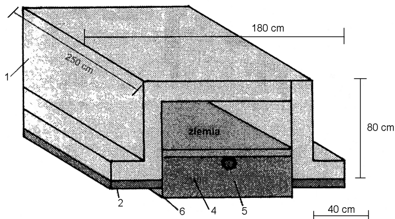
Rys. 2.1. Schemat konstrukcyjny przejścia dla płazów i gadów
